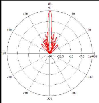
E-Plane
